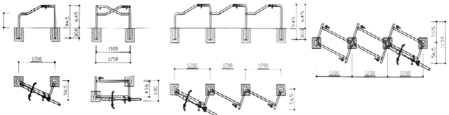
ALPHA-Reihenanlage doppelseitig
